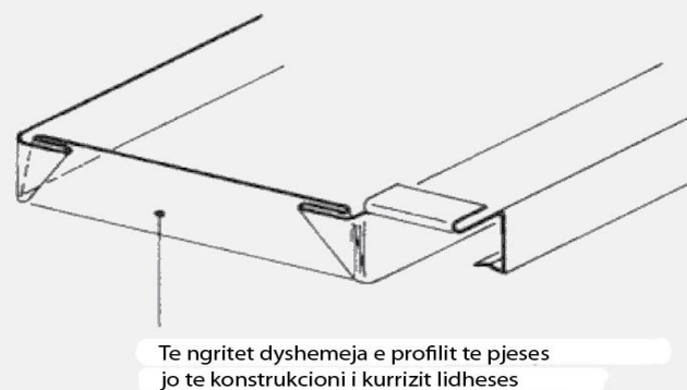
Fig. 12 Konstruksioni i uji kthyesit
