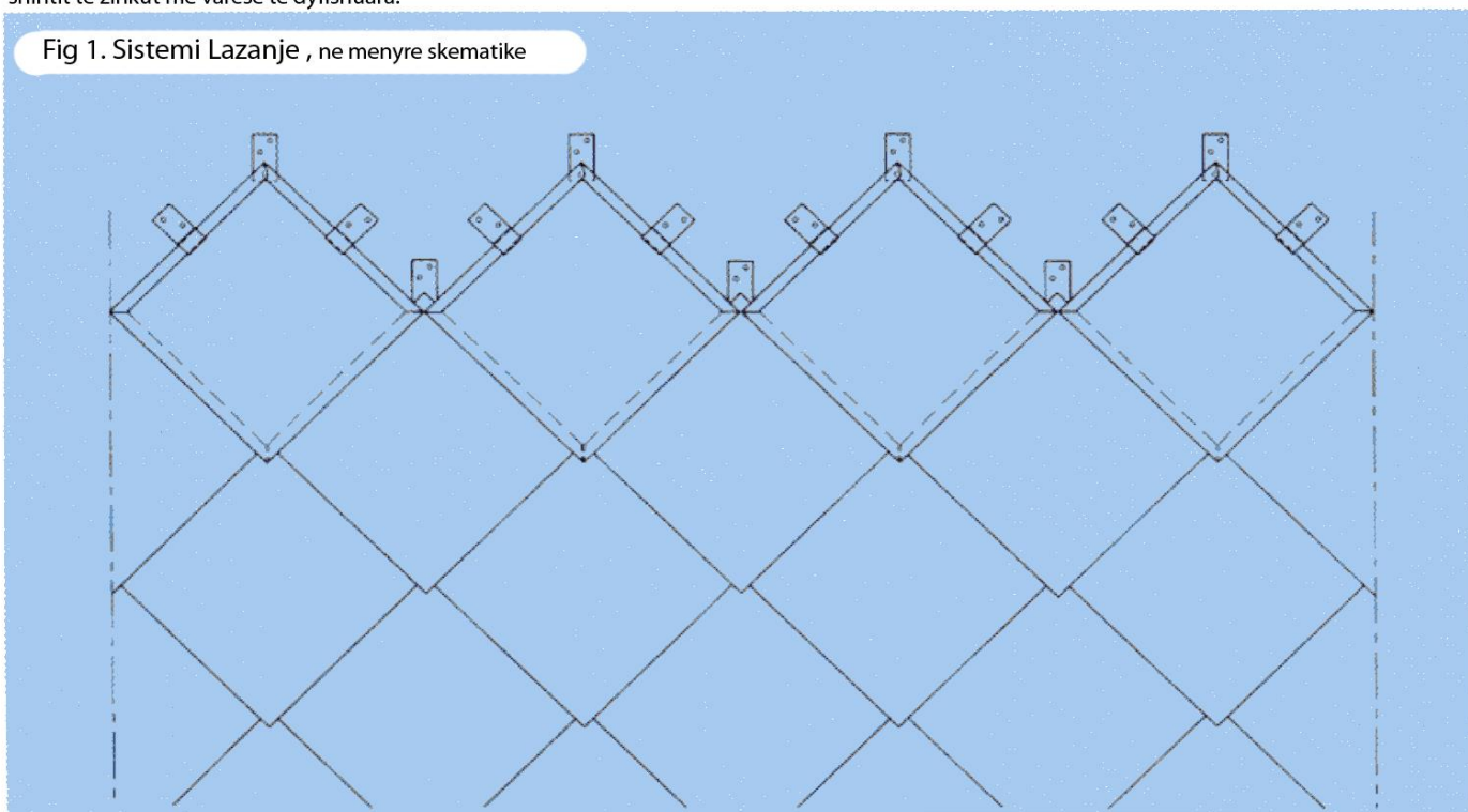
Fig. 2 Lazanje katerkendeshe (katrore)
