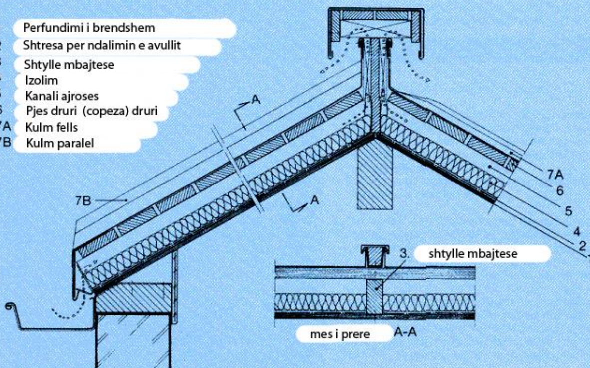
Fig. 1.: Konstrukcioni -- ndertimi i kulmit te izoluar
