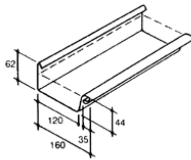
Përmaset e ullukut B30
