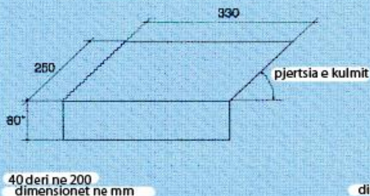
Fig. 9 Lidhja (mbyllja) nen a, detajet e pjeses kulmit
