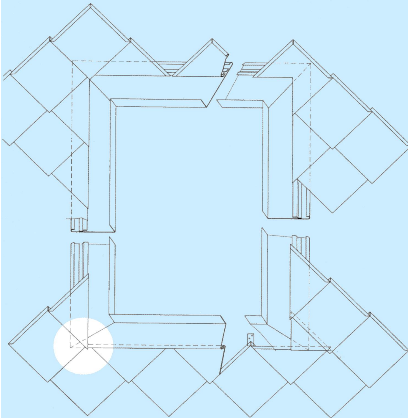
Fig. 14 Kulm i nderprere
