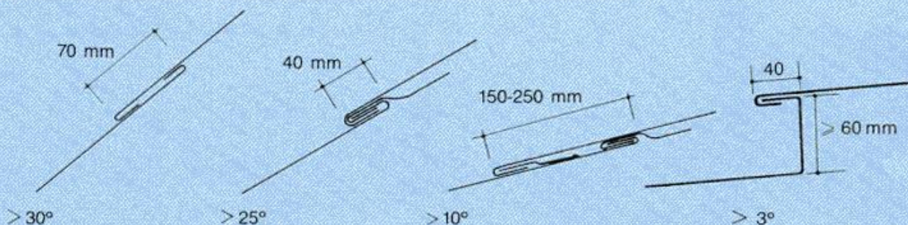
Fig. 8 Metodot e lidhjes tek bashkimet anesore te pjeseve fellse
