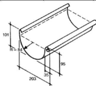
Përmasat e ullukut M37
