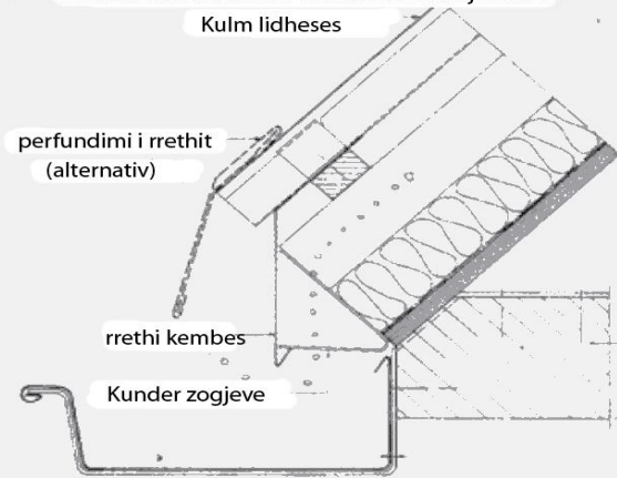
Fig. 15 Konstruksioni kembesor i kulmit me u.drejt kendesh
