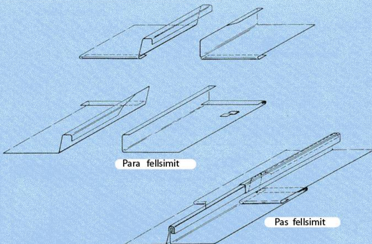
Fig.9 Bashkimi i fellsave tek lidhja e pjeseve fellse
