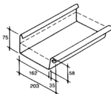
Përmasat e ullukut B37
