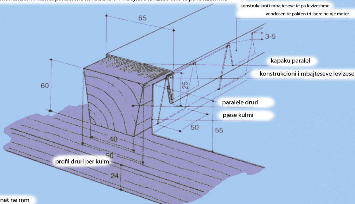
Fig. 3 Sasia e mbajtesëve ne m 2 dhe hapsira e tyre ndermjet, m'varesisht prej gjersis se pjeseve dhe lartesis se kulmit.
