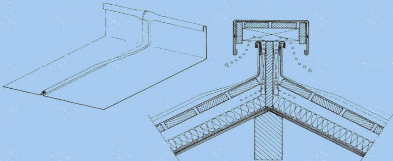
Fig. 13 Lidhja (mbyllja) e kurrizit me fells te rrahur rrafsh.
