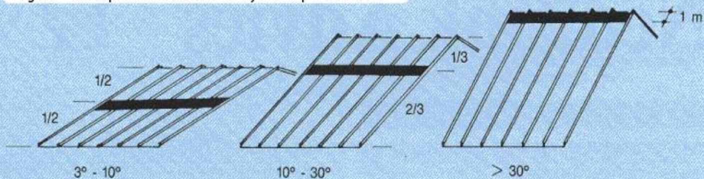
Fig. 11 Vendi per konstrukcionet e mbajtseve te pa levizeshme.
