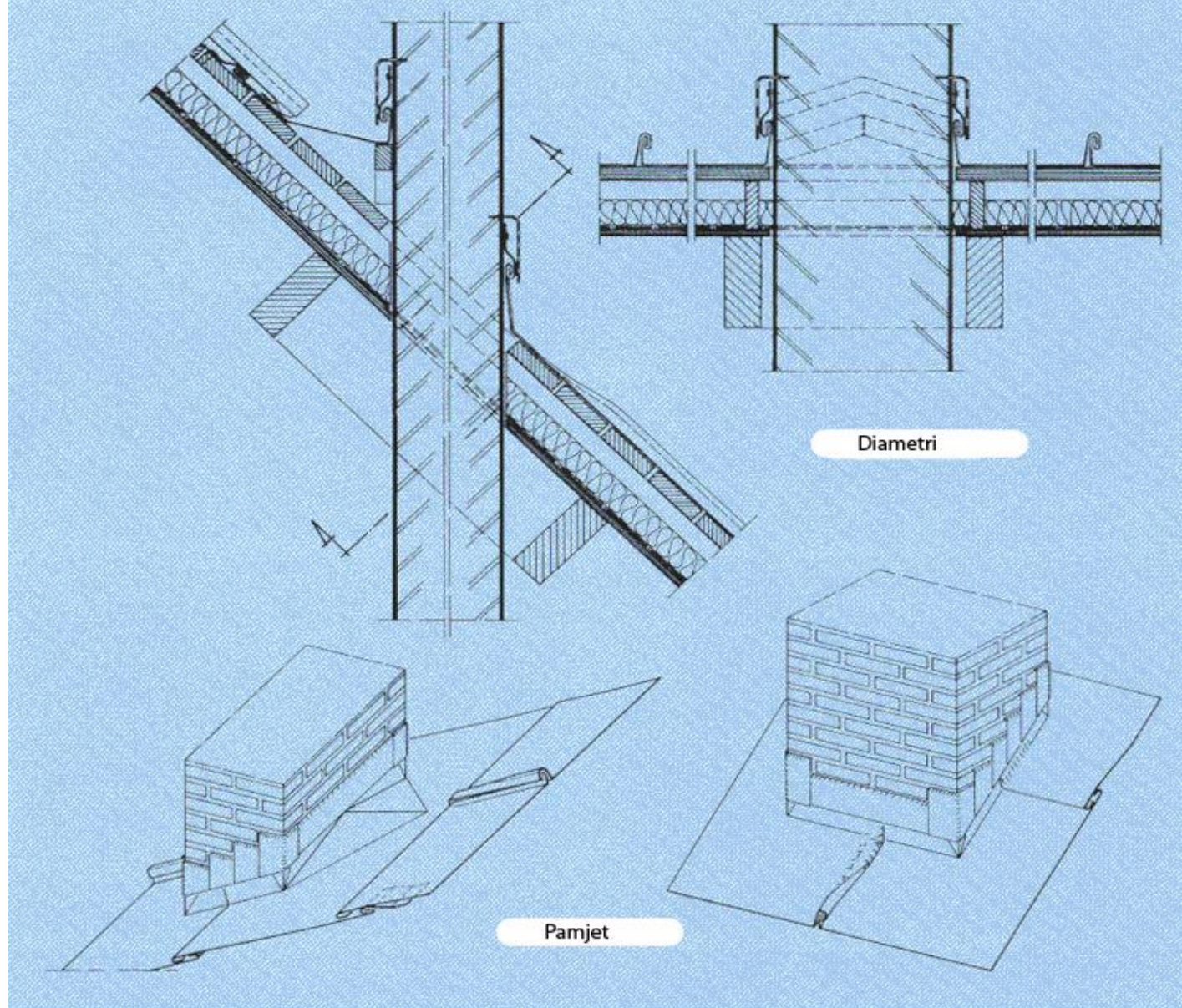
Fig. 17 Nderprerjet e kulmit
