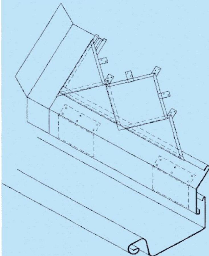
F.13 Lidhja e nje kendi druri qe bashkon 2 pjes kulmi
