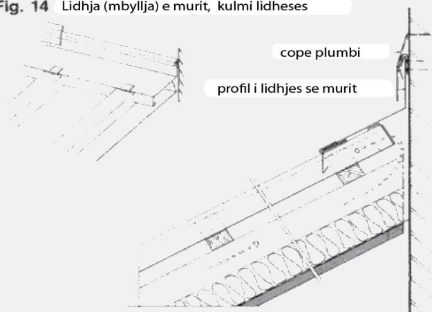
Fig. 14 Lidhja (mbyllja) e murit, kulmi lidhese
