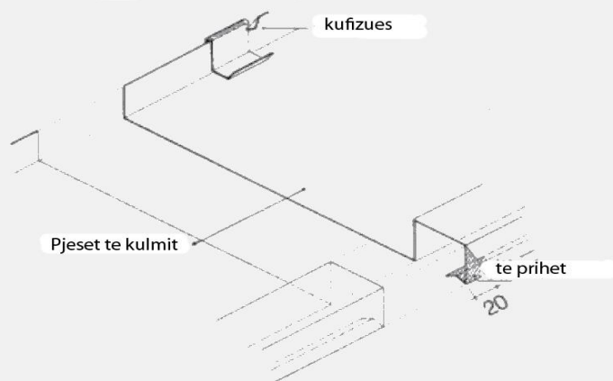
Fig. 11 Ngjitja e copeve te pjeses te saldoen bashk
