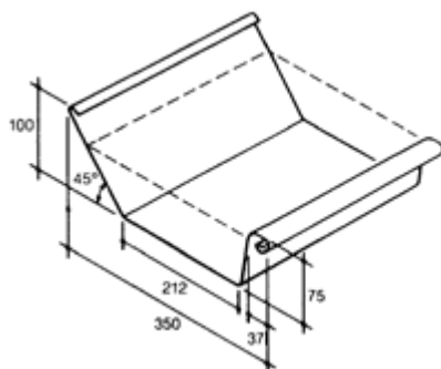
Përmasat e ullukut B50
