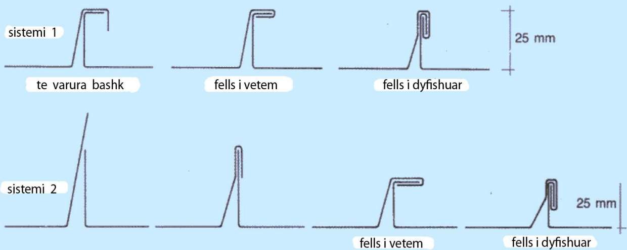
Fig.2 lidhja (bashkimi) fellsave
