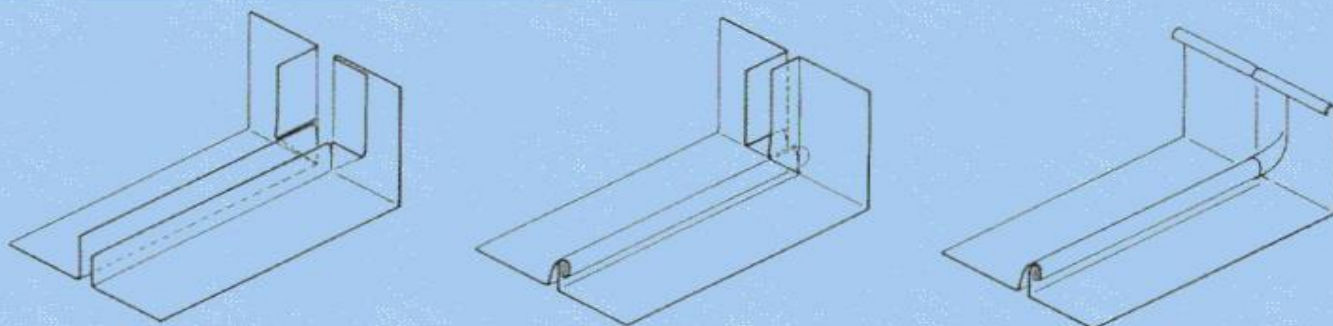
Fig. 14 Lidhja (mbyllja) e kurrizit sipas metodes palosese.
