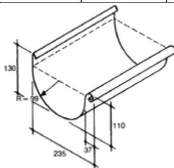
Përmasat e ullukut M44
