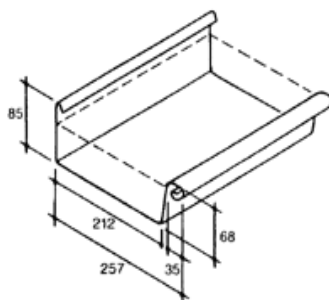
Përmasat e ullukut B44
