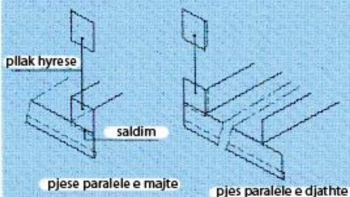
Fig. 9 Lidhja (mbyllja) nen a, detajet e pjeses kulmit
