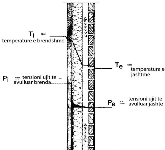
Fig. 2 Rritja e temperaturës dhe tensionit ujit të avulluar tek një konstrukcion i ventiluar.
