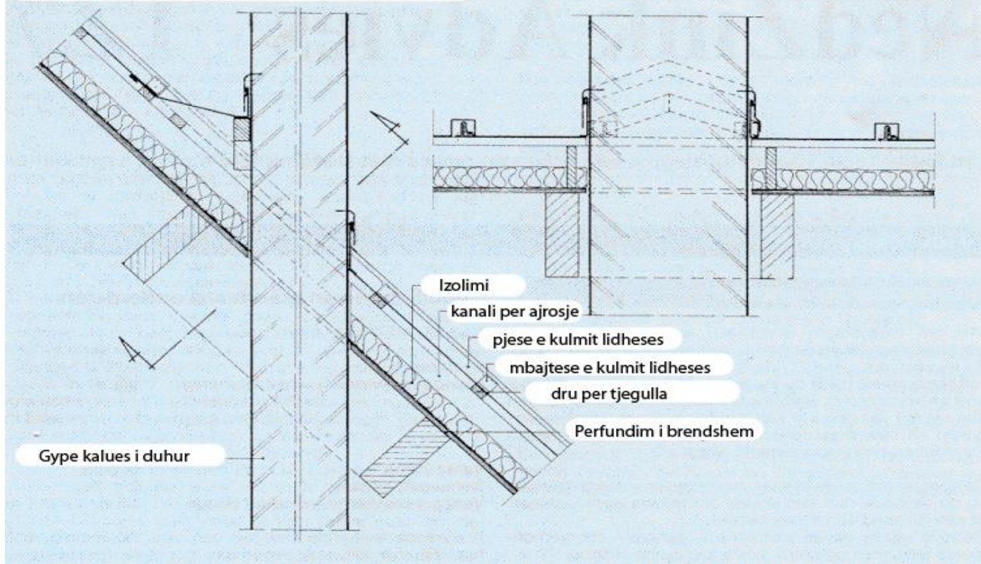
Fig.16 Konstruksioni i gypit kalues neper mes te kulmit
