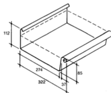
Përmasat e ullukut B55
