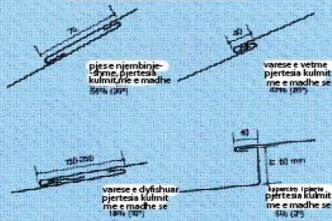
Fig. 10 Metodat e lidhjes tek nyjet e paraleleve
