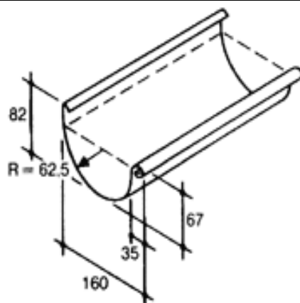
Përmasat e ullukut M30
