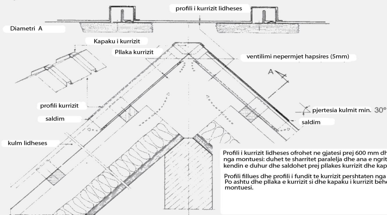
Fig. 13 Konstruksioni i kurritzit lidhese
