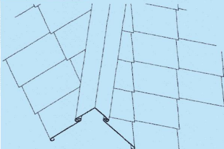
F.13 Lidhja e nje kendi druri qe bashkon 2 pjes kulmi
